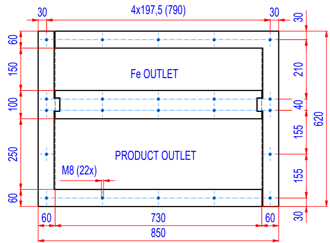
BOTTOM FLANGE
