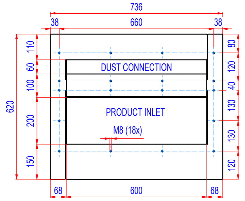
TOP FLANGE
